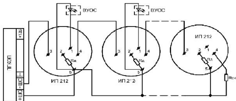
Рис.3 Схема подключения извещателей
