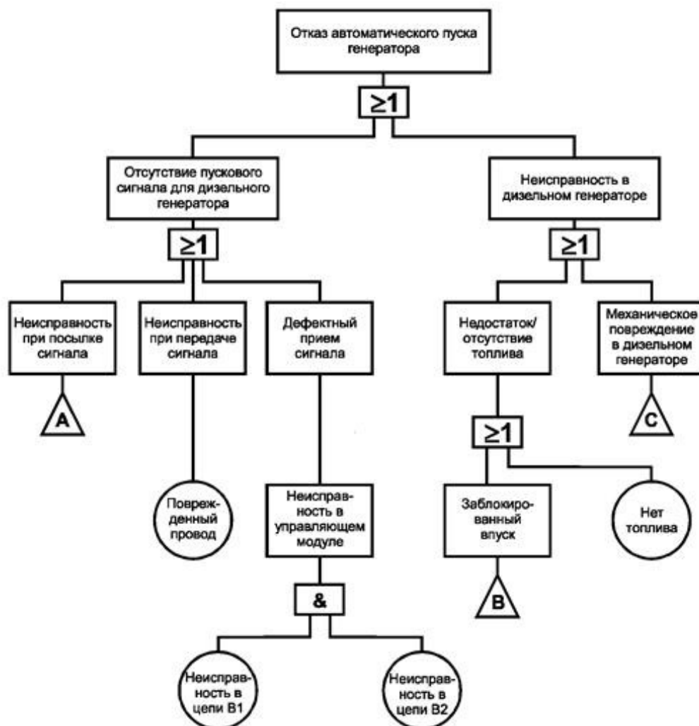
Рисунок А.1. Пример "дерева неисправностей"
