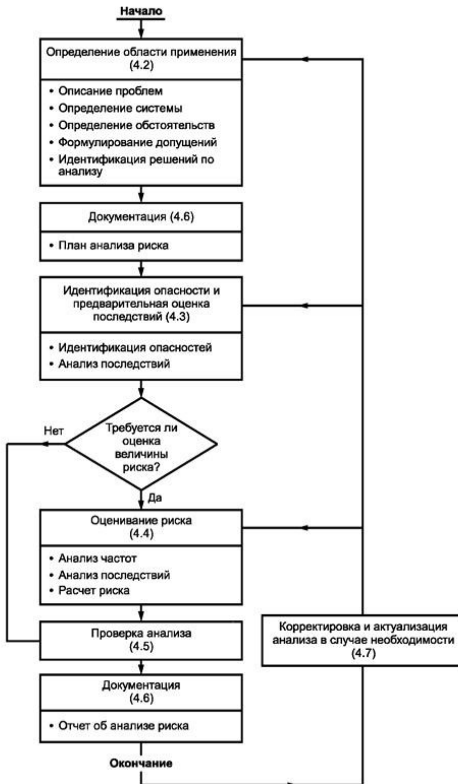
Рисунок 2. Процесс анализа риска (раздел 4)
