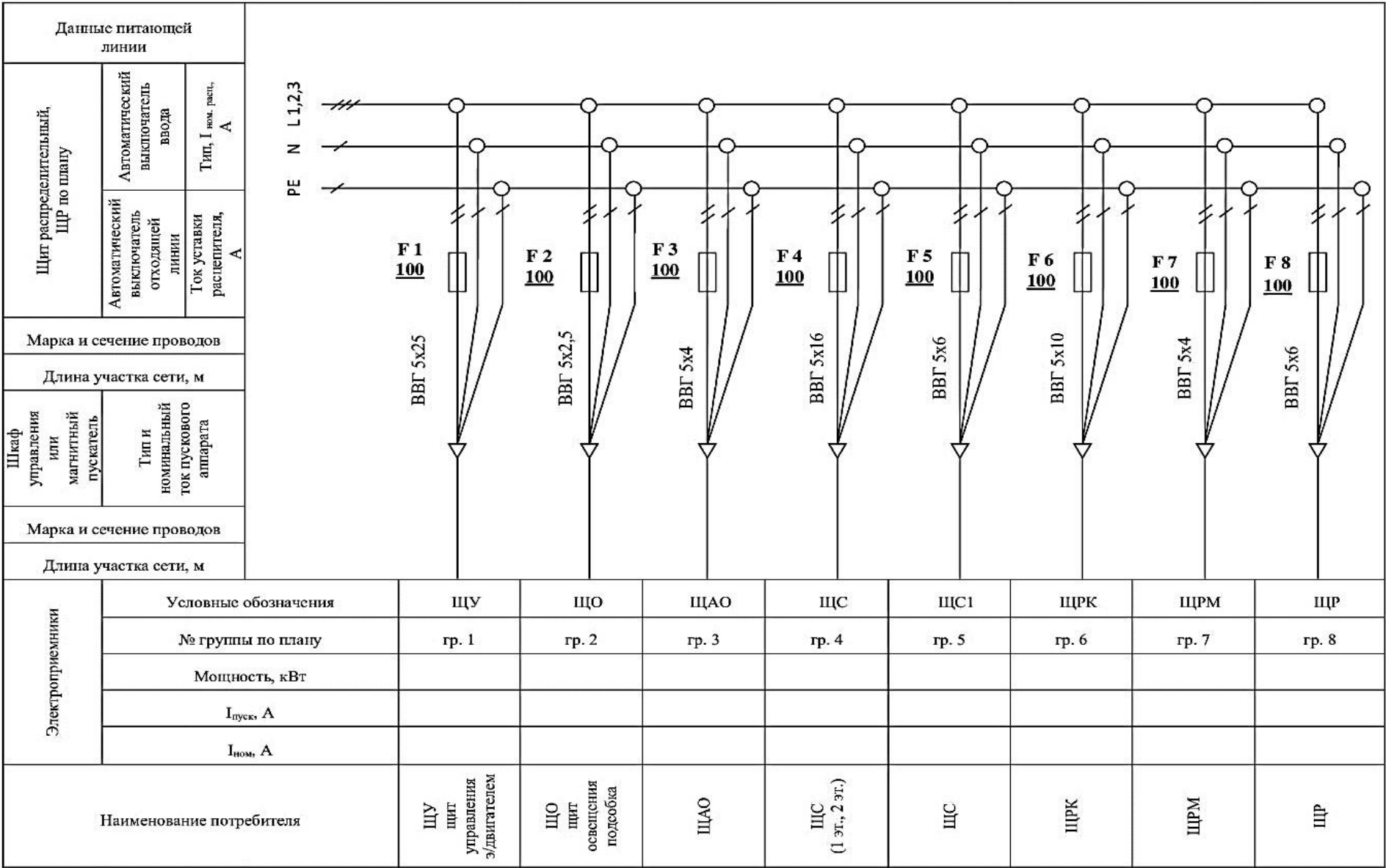
Однолинейная схема шкафа с предохранителями
